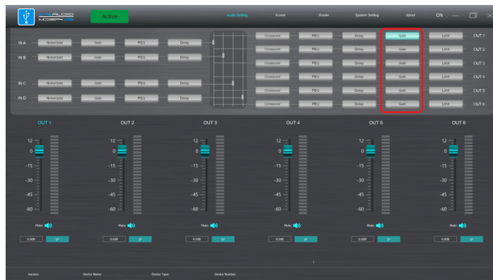
Настройка уровня выходящего сигнала и MUTE для OUTPUT 1/2/3/4/5/6.
